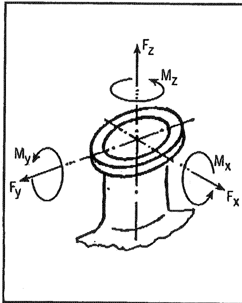
Kräfte / Drehmomente
